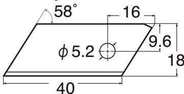
Ersatzklinge BZL11P, Detailsicht
