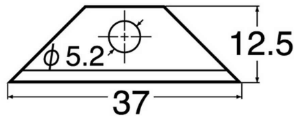
Vue détaillée BR-400P
