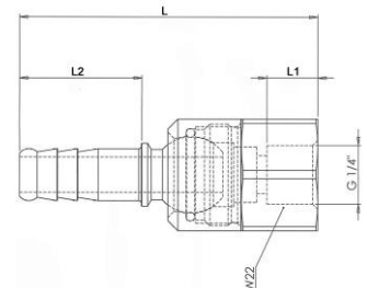
Schlauchtülle, Innengewinde
