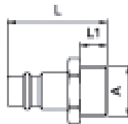
Nippel Außengewinde
