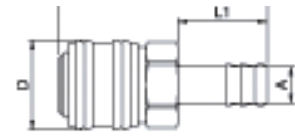
Schlauchtülle
