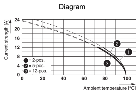
Type: GMSTB 2,5/...-ST-7,62 with GMSTBA 2,5/...-G-7,62
