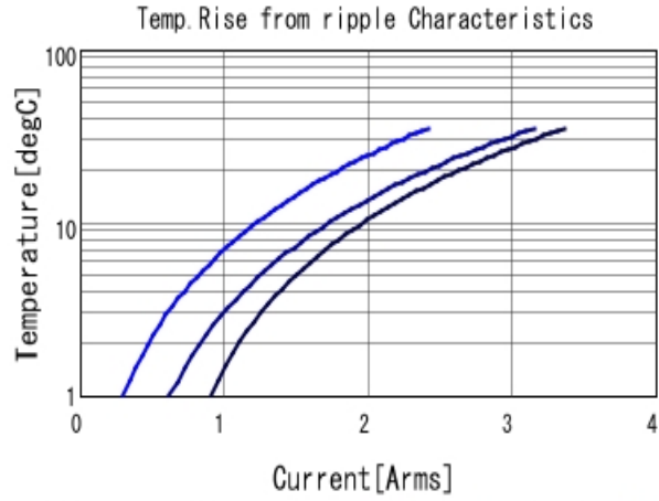
GRM033R61A225KE47 Temp. rise ■ 100kHz ■ 500kHz ■ 1MHz
