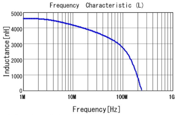
■ LQW32FT4R7M0H L
