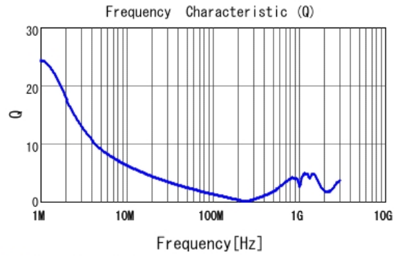
■ LQW32FT4R7M0H Q
