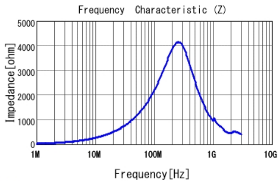
■ LQW32FT4R7M0H |Z|
