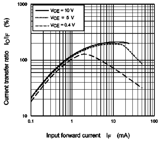
Fig. 11.10 I_C/I_F - I_F
