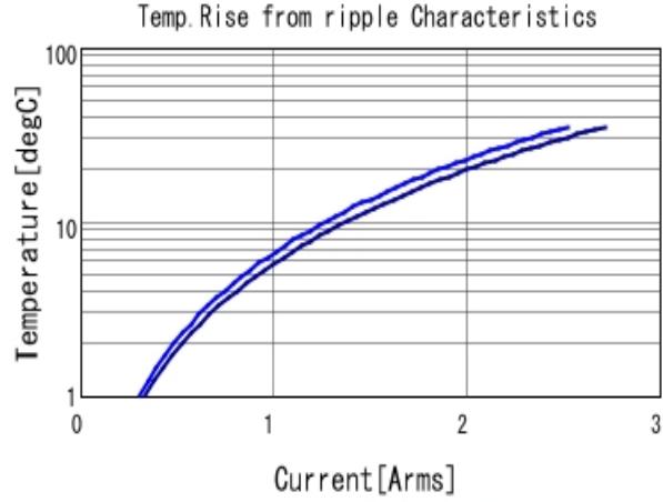
GCJ188R71E105KA01 Temp. rise ■ 500kHz ■ 1MHz
