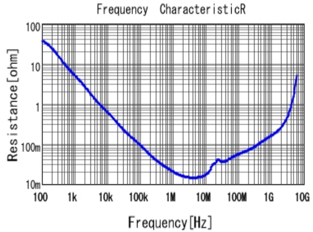
■ GCJ188R71E105KA01 R DCOV, 25degC
