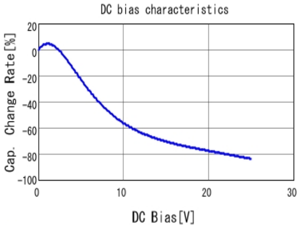
■ GCJ188R71E105KA01 C-DC bias capchange, 25.0degC, AC1.
