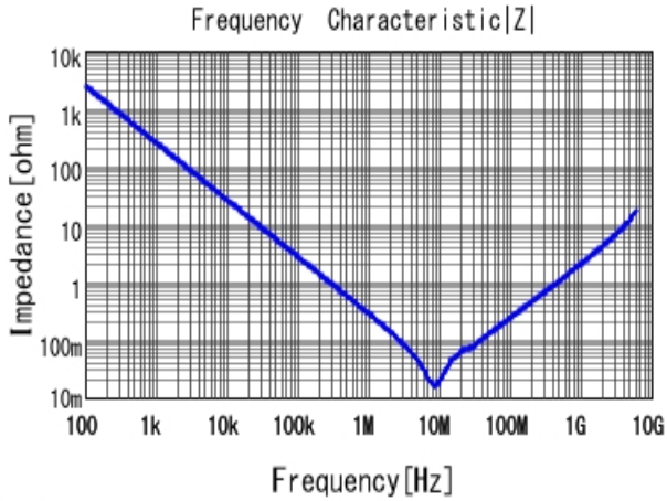
■ GCJ188R71E105KA01 |Z| DCOV, 25degC
