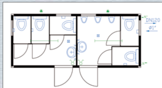
Grundriss-Beispiel 20' WC-Container D/H
