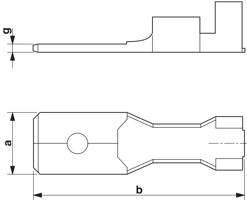
Maßzeichnung
