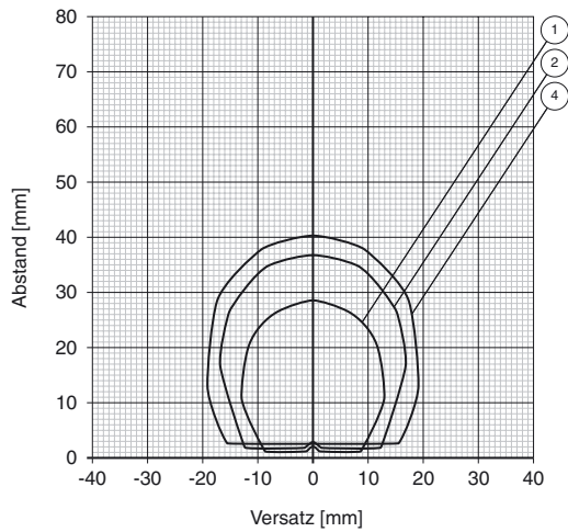
Lesebereich auf Aluminium IPC02-16
