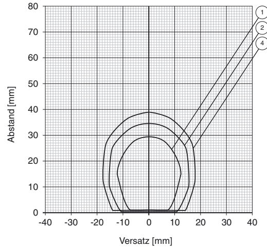
Leseabstand auf Stahl IPC02-16
