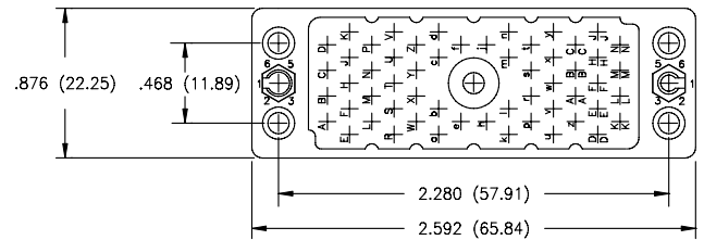
56 PIN RECEPTACLE
