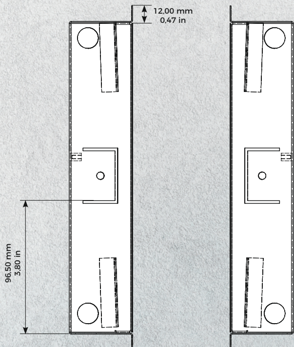
Montagerückgehäuse
