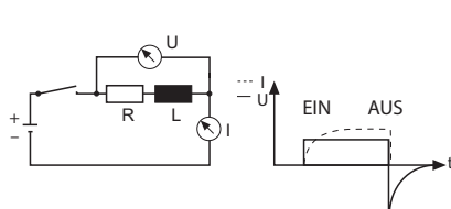
Strom-/Spannungsverlauf beim Schalten einer Relaispule Abb.2
