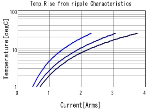
KRM55TR72E225MH01 Temp. rise ■ 50kHz ■ 100kHz ■ 300kHz
