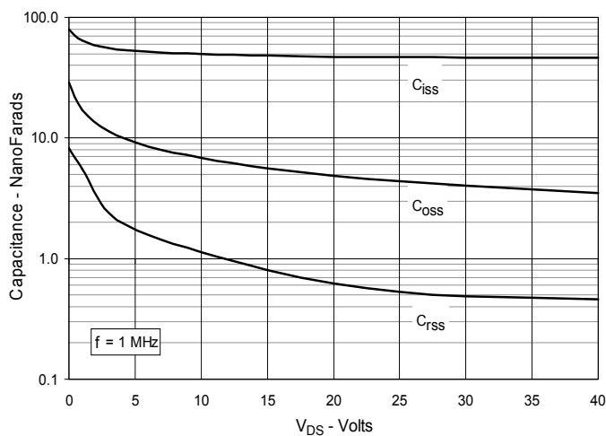
Fig. 11. Capacitance
