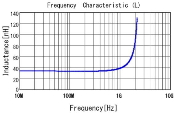
■ LQW2BAS33NG00 L
