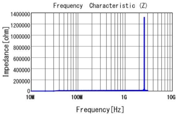
■ LQW2BAS33NG00 |Z|
