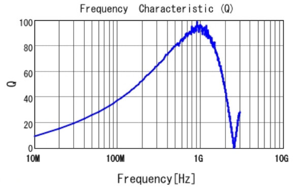
■ LQW2BAS33NG00 Q
