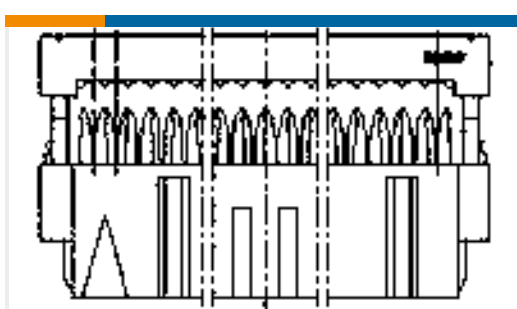
TE Teilenummer6-215915-0 AMP-LATCH 15.2 HIGH TAPE
