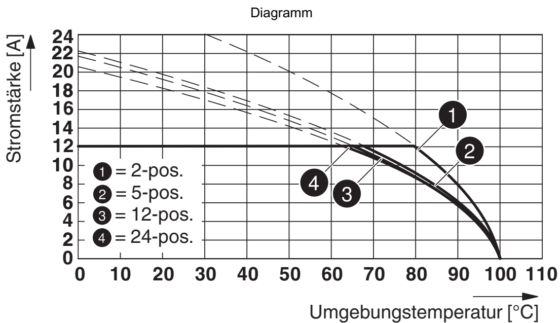
Typ: MSTB 2,5/...-ST-5,08 mit MSTB 2,5/...-G-5,08
