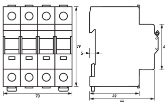
Maßzeichnung Gruppenansicht
