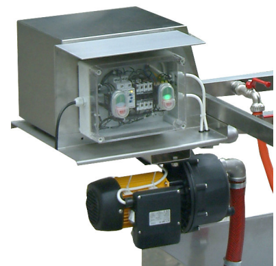
Ausführung HT-304-A
