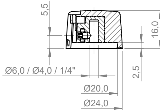
Schnitt A-A
