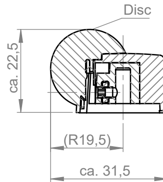
Schnitt A-A
