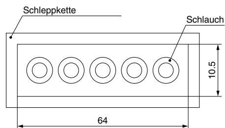
Schlauchabmessungen im Inneren der Schleppkette
