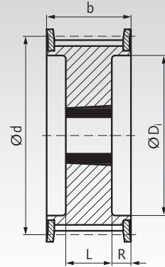
Ausführung 18F
