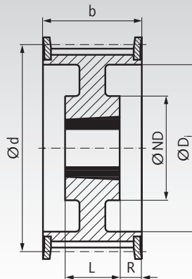
Ausführung 19F
