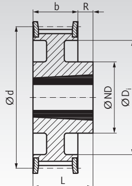
Ausführung 11F
