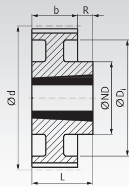
Ausführung 11
