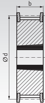
Ausführung 15F
