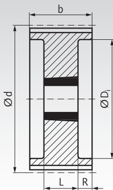
Ausführung 18
