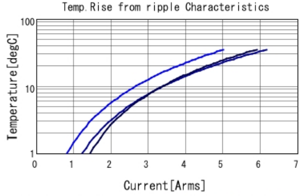
GRM32EC72A106KE05 Temp. rise ■ 80kHz ■ 400kHz ■ 800kHz
