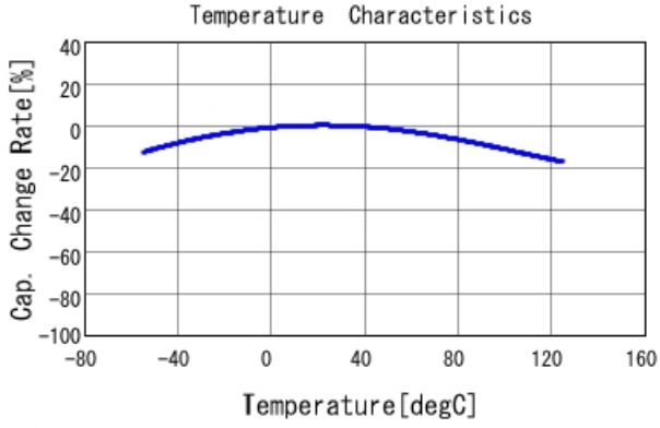
■ GRM32EC72A106KE05 C-Temp. capchange, DCO. 0V, ACO. 1Vrm
