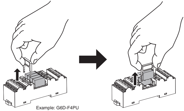
Example: G6D-F4PU
