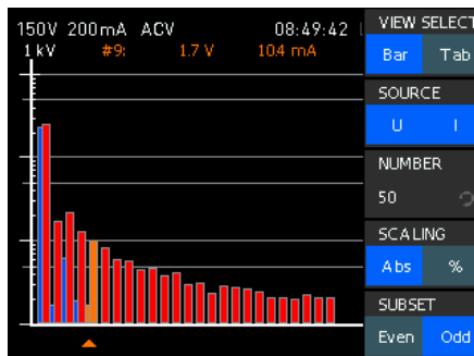
Harmonischen-Analyse: Balkendiagramm
