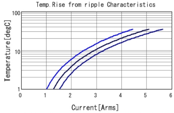
GRM31CR71H475KA12 Temp. rise ■ 100kHz ■ 500kHz ■ 1MHz
