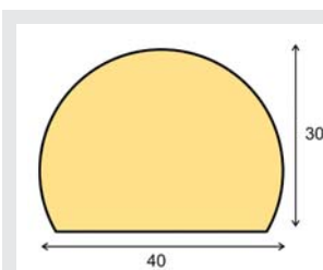
Flächenschutz Kreis, Typ C
