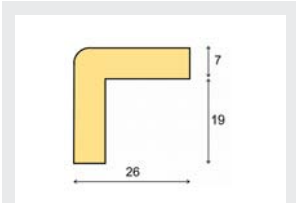
Kantenschutz Winkel, Typ E
