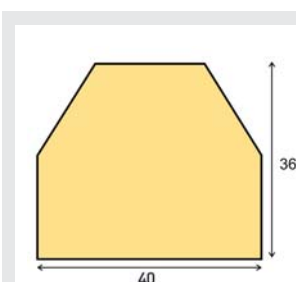
Flächenschutz Trapez, Typ CC
