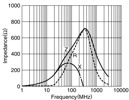
MMZ0603S471C
