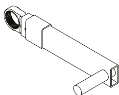
Gleitzapfen (versch. Längen möglich)
