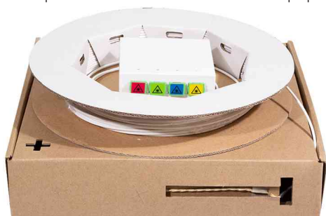
Visuel de référence : Boîte d'épissure FTTH avec câble d'installation, 4x SC / APC
