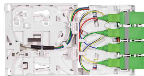
Visuel de référence : Boîte d'épissure FTTH avec câble d'installation, 4x SC / APC
