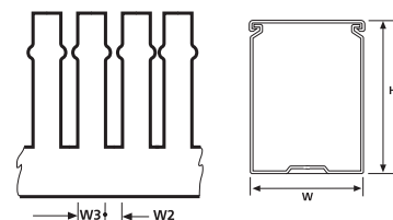
T1E kabelkanal
