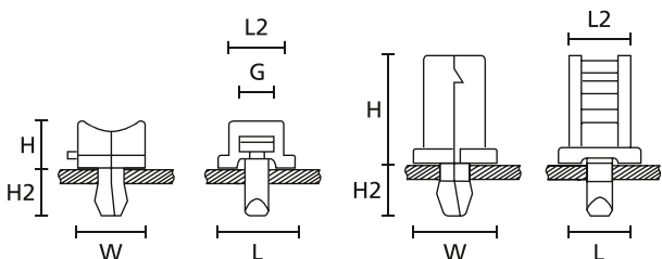
Keilsockel TY5K2
