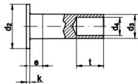
Form B = Halbhohl-Niete
