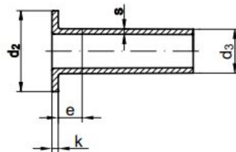
Form C = Hohl-Niete
