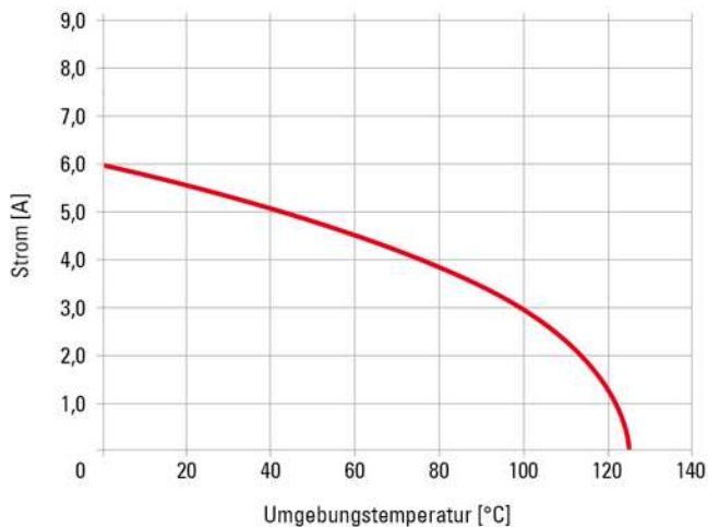
Stromtragfähigkeit Signalkontakte
