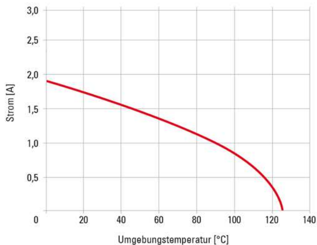
Stromtragfähigkeit Signalkontakte
