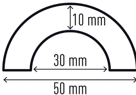
Vue détaillée: profilé de protection pour tubes P30
