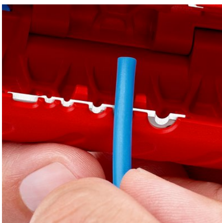
90 22 02 SB: El dispositivo práctico de posicionamiento facilita la colocación de conductores individuales para pelar
