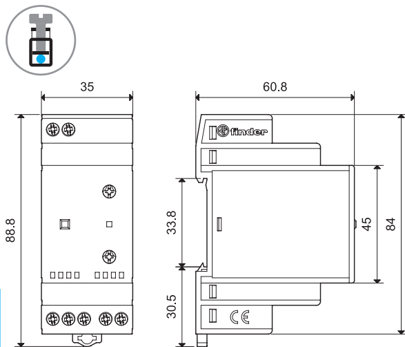
11.41 Schraubklemmen
