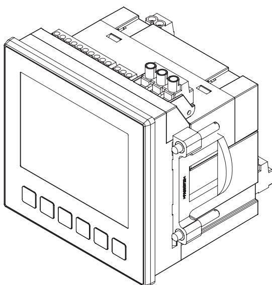
Ansichten des Messgeräts UMG 96-PA/96-PQ-L mit aufgestecktem Modul 96-PA-RCM-EL
