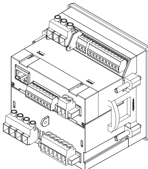
Ansichten des Messgeräts UMG 96-PA/96-PQ-L mit aufgestecktem Modul 96-PA-RCM-EL
