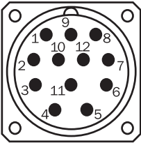
Ansicht Gerätestecker M23 an Leitung/Gehäuse
