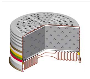
Dräger Filter Rd91: Schnittzeichnung
