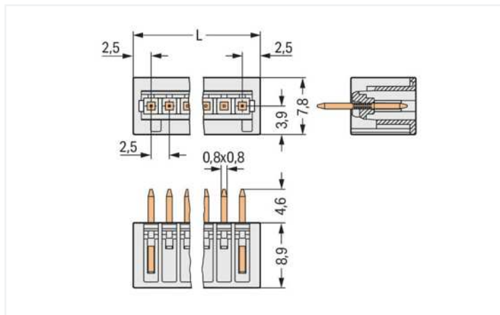
Abmessungen in mm L = (\text{Polzahl} + 1) \times \text{Rastermaß}
