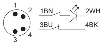
Abb. 8 1 NO + 1 NC (mit LED)
