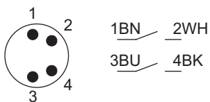
Abb. 5 2 NO (ohne LED)
