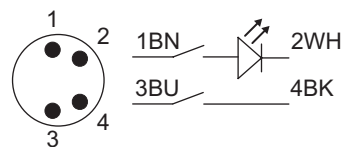
Abb. 6 2 NO (mit LED)
