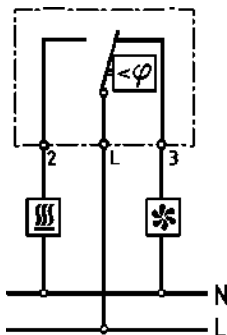
Anschlussdiagramm
