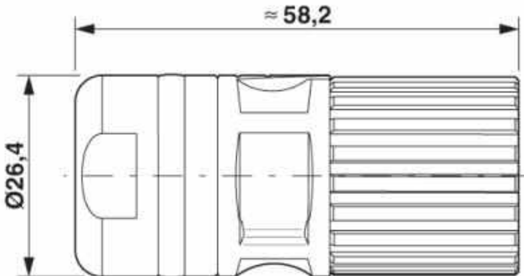
Maßzeichnung
