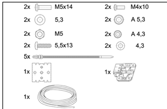
Рис. 1: Прилагаемые комплектующие
