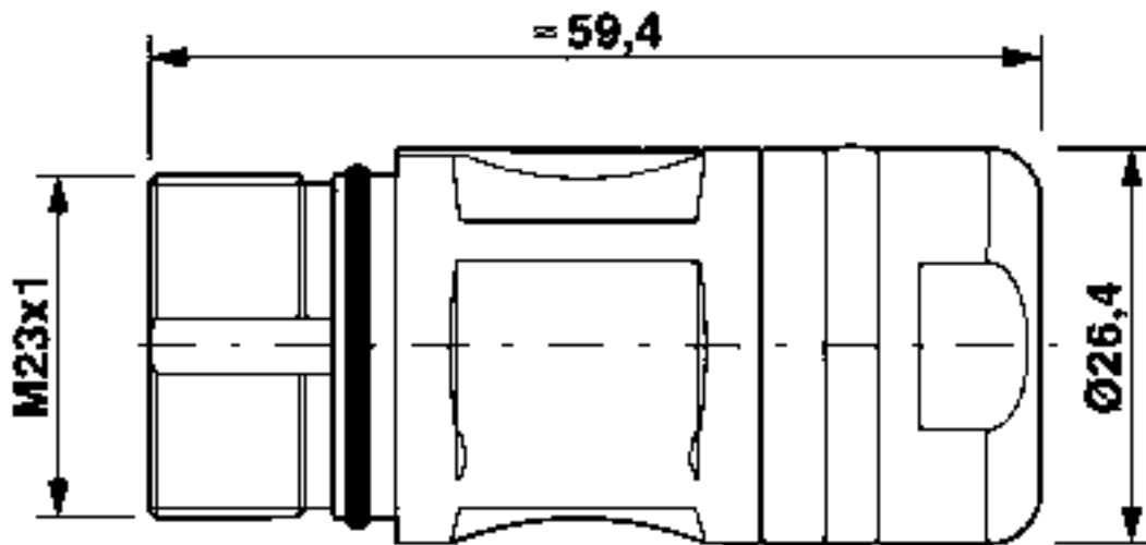
Maßzeichnung
