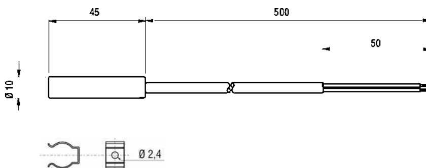
Befestigungsclip, Art. Nr. 09008.0-01 (1 VE = 2 Stück)
