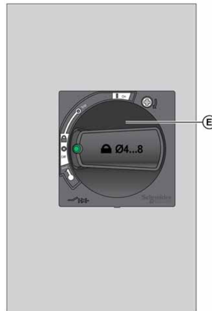
Schaltschranktür geschlossen
