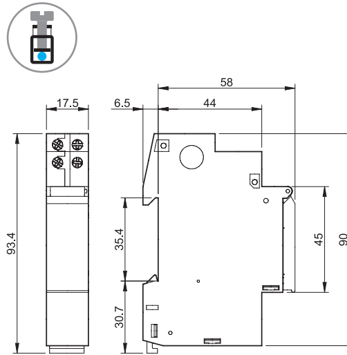
12.11 Schraubklemmen
