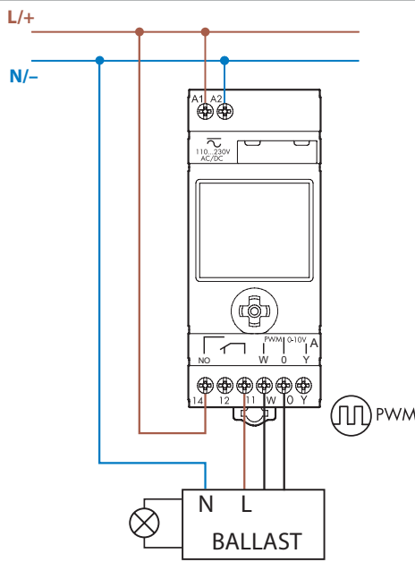
Typ 12.A4
