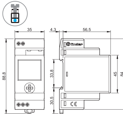
12.51/12.81 Schraubklemmen
